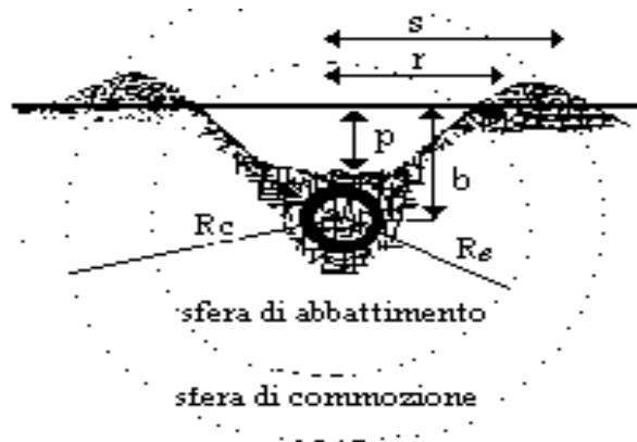
Elementi di cratere (o imbuto) creato da una carica concentrata
